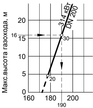
Необходимый общий напор горелки, Па
